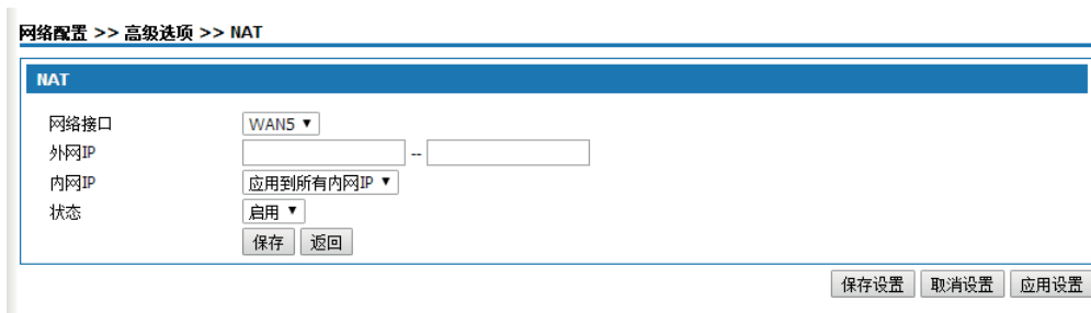
图5-16 添加NAT设置
