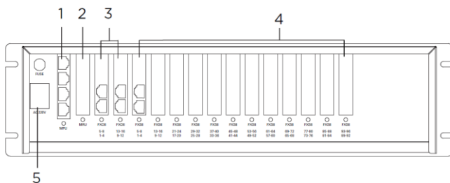
图1-5 HB300 前面板图
