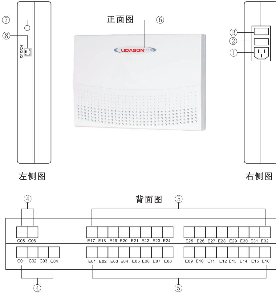
2外线8分机至6外线32分机设备连接图三：
